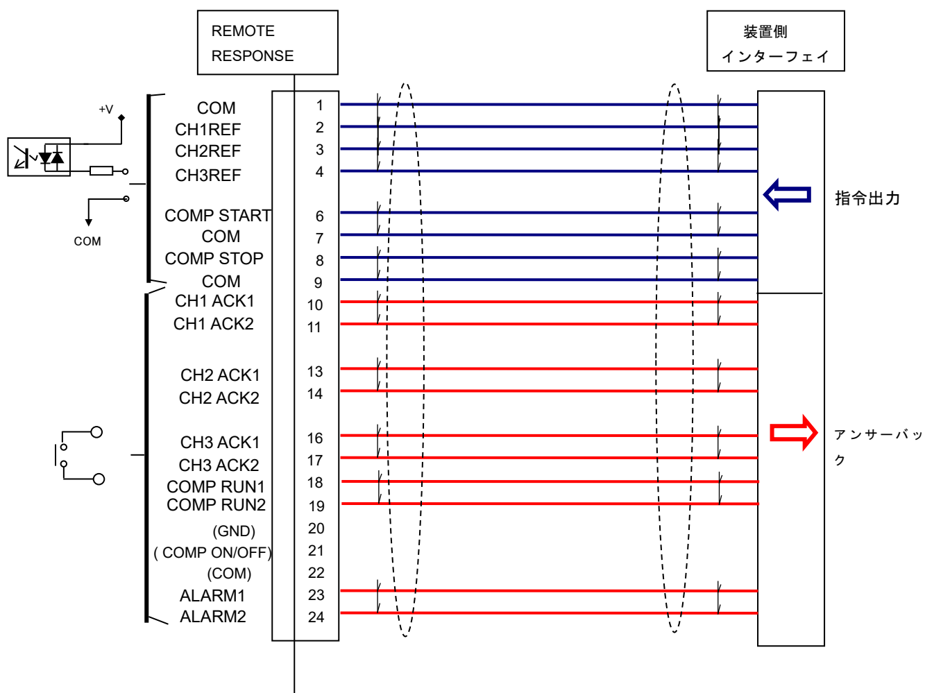
図 4-11 (C30MVR) 複数クライオポンプ運転のための「モメンタリ操作モード」配線例
