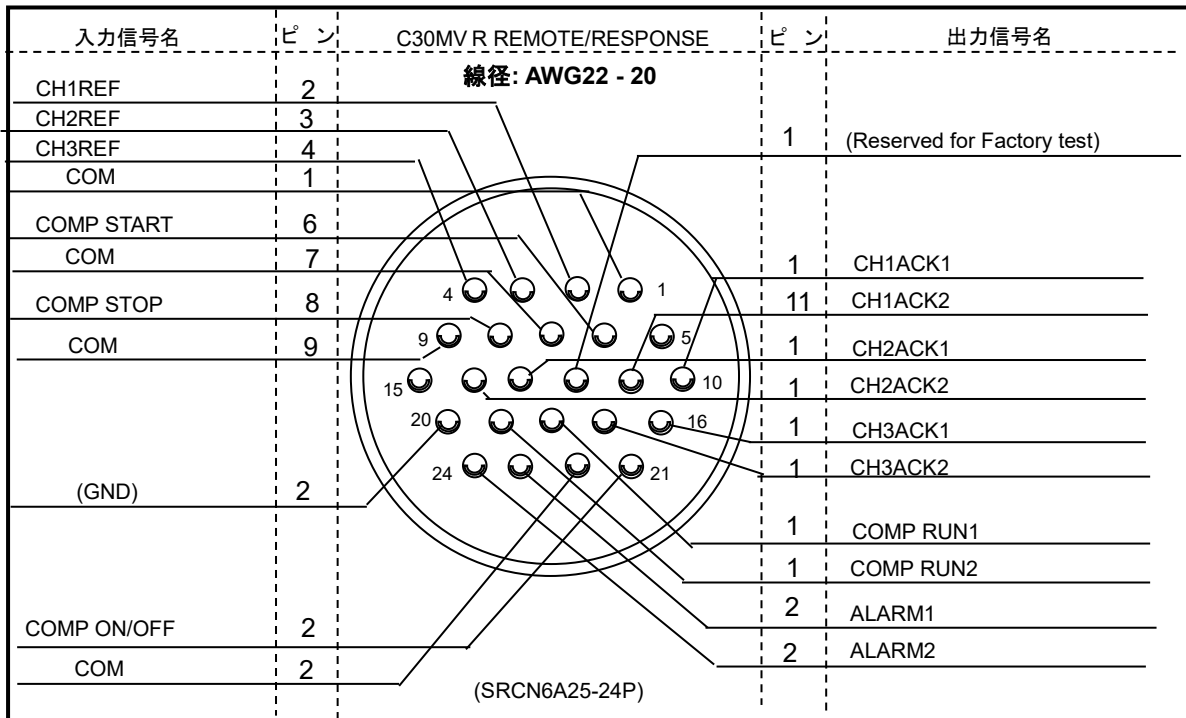
図 4-9 C30MVR 用リモートコネクタピン定義(プラグ半田付け側から見て)
