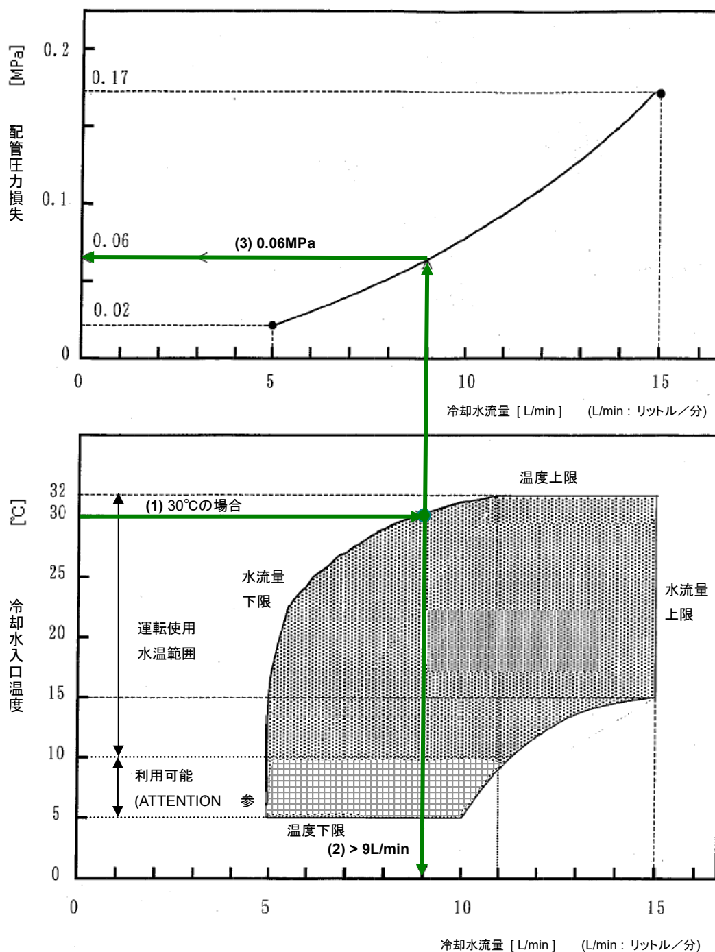
図 2-4 冷却水流量と冷却水入口温度、配管圧力損失(適用:C30PV RT)
