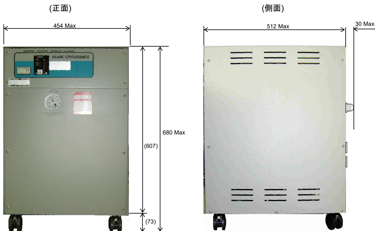
図 1-5 C30VR コンプレッサの外形寸法
