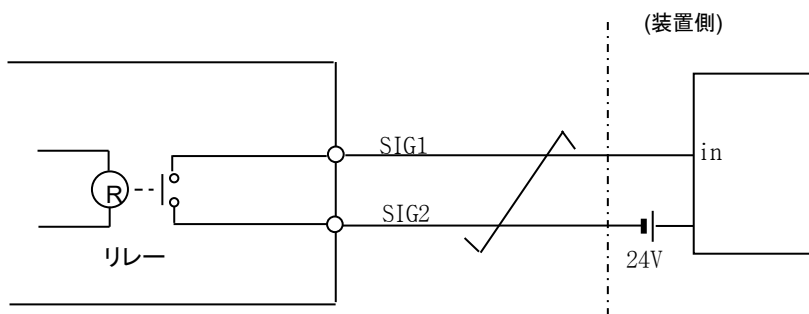
図 2-6 リモート出力インターフェース回路
