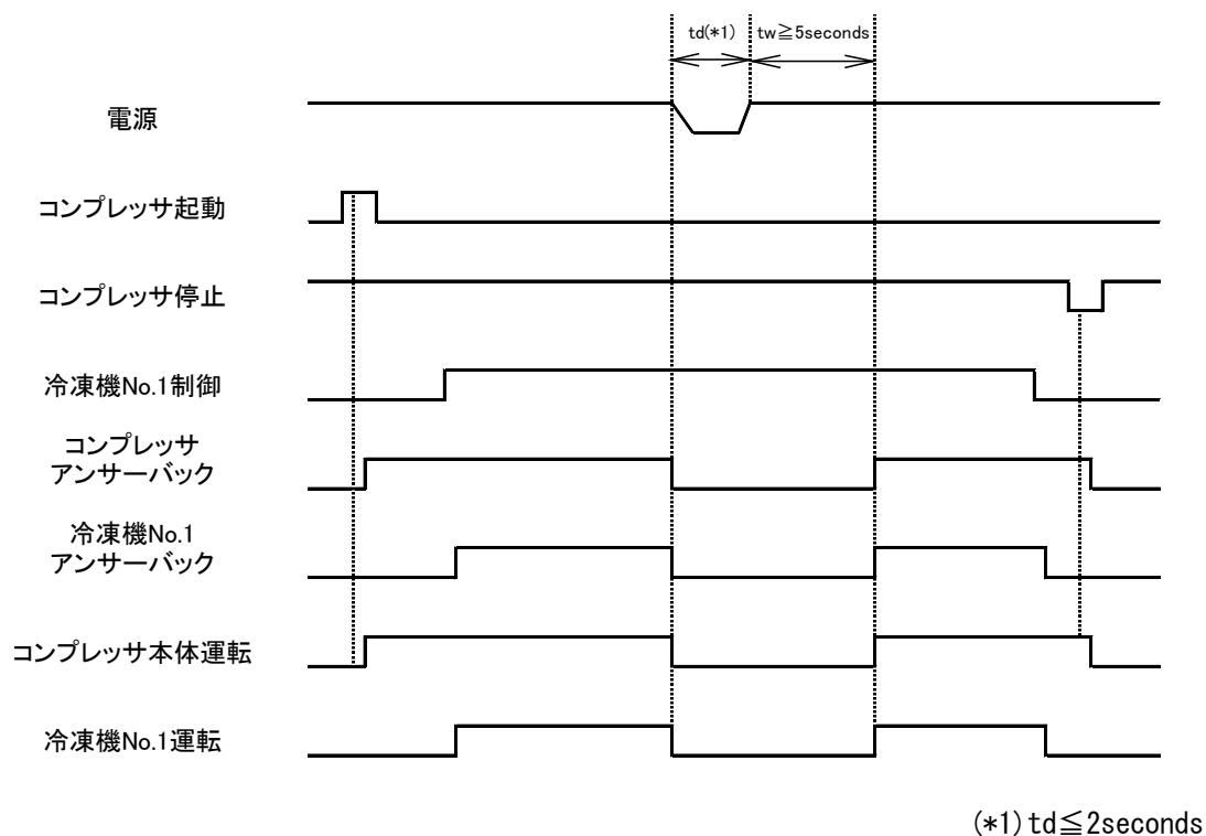
図 2-11 瞬停時の C30VR のタイムチャート (モメンタリ操作モードの場合)
