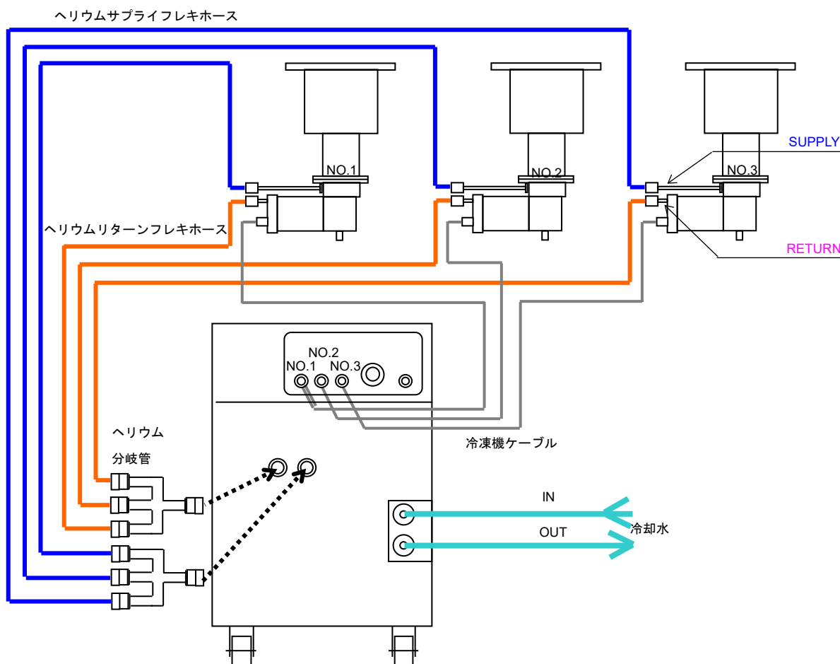
図 4-6 複数台のクライオポンプとコンプレッサの接続（2台の場合）
