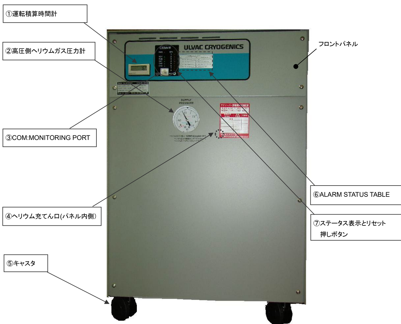
図 1-6 コンプレッサ正面
