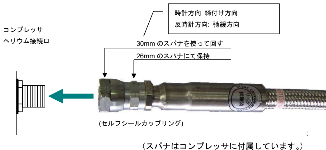
図 4-4 コンプレッサと冷凍機に対するフレキホースの取付け、取り外し
