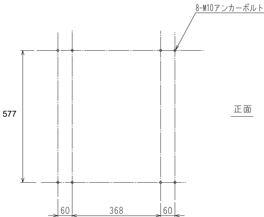
図 1-8 アンカーボルト固定位置 (例)
