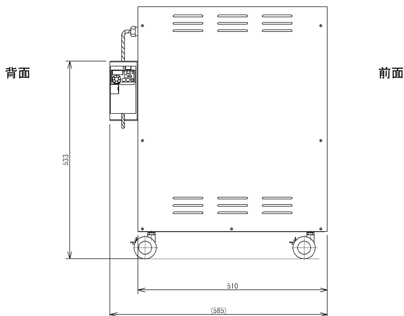
図 1-10 インバータ搭載 C30VR コンプレッサ
