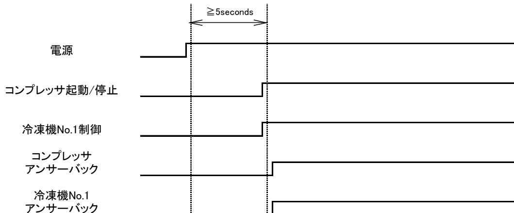
図 2-9 電源投入時の信号の遅れ（オールタネート操作モードの場合）
