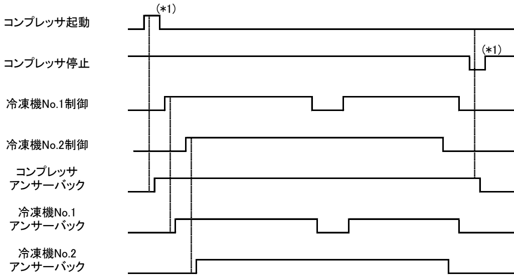
図 2-8 2 台の冷凍機の運転を「モーメンタリ操作モード」で行う場合のタイムチャート
