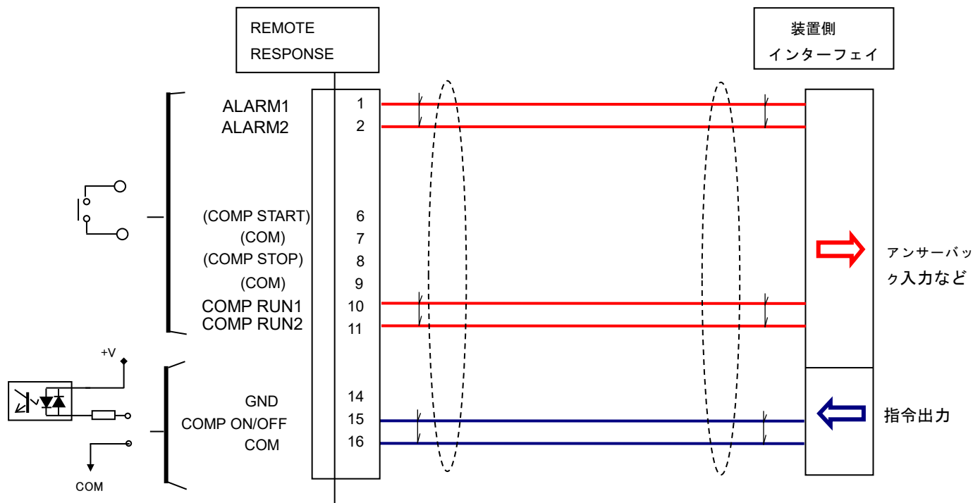
図 4-10 (C30VR) 1 台のクライオポンプ運転のための「オールタネート操作モード」配線例
