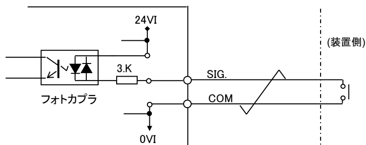
図 2-5 リモート入力インターフェース回路
