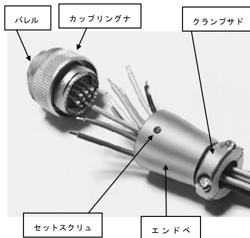
図 4-12 コネクタ各部の名称
