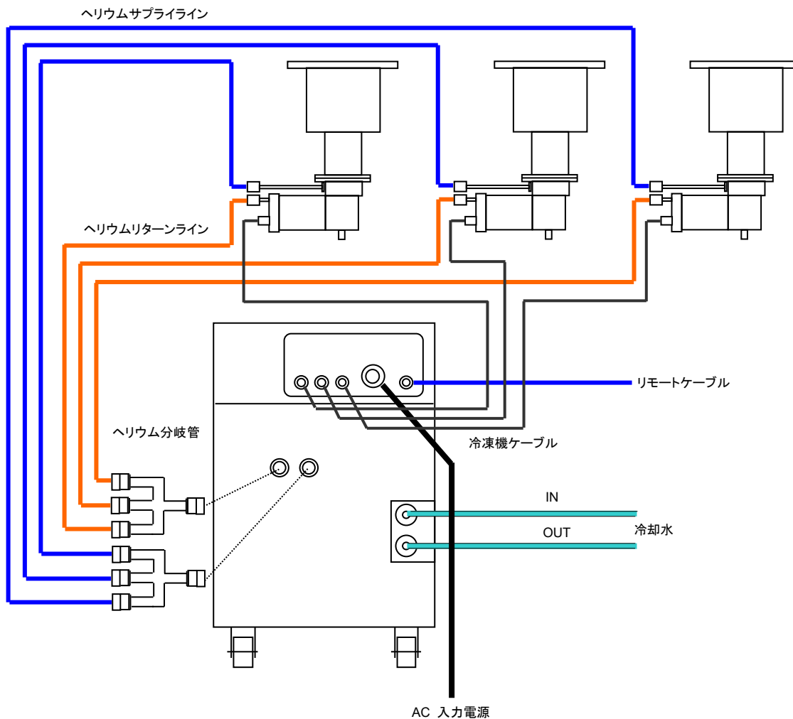
図 1-9 クライオポンプと C30MVR コンプレッサの接続
