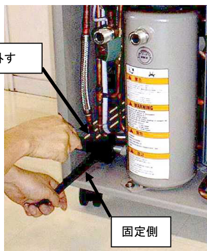
図 7-1 ヘリウムガス接続口のナット2個を外す(左)
