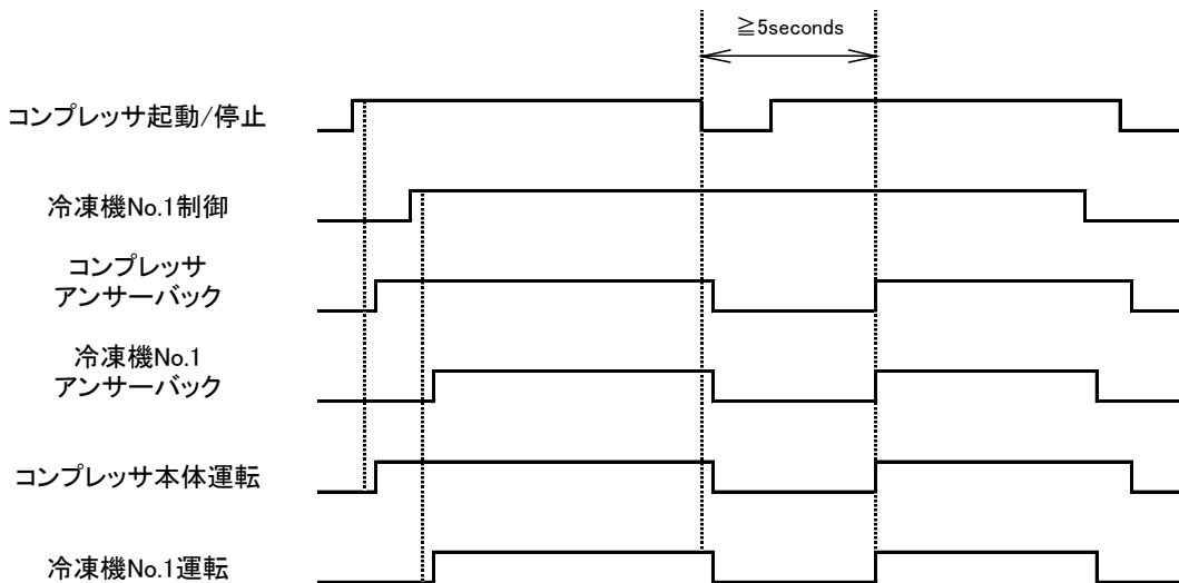
図 2-10 停止から起動までの時間が短かった場合の信号遅れ (オールタネート操作モードの場合)
