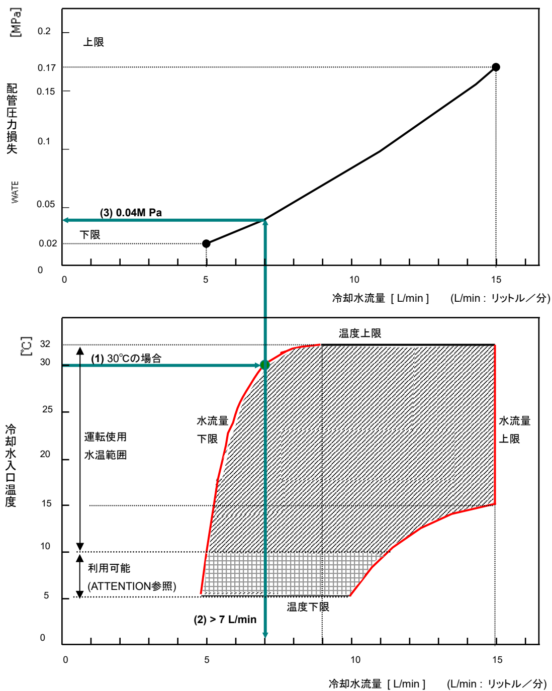
図 2-3 冷却水流量と冷却水入口温度、配管圧力損失(適用:C30PV RT 以外)
