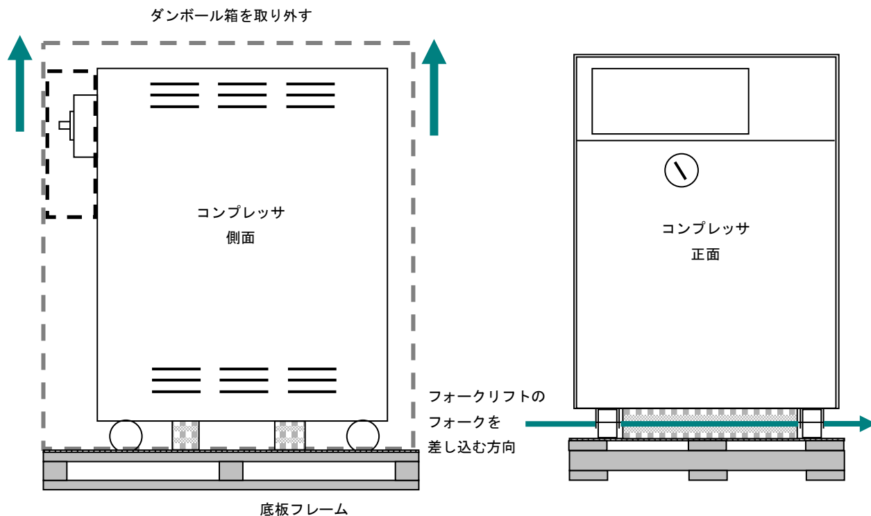
図 3-2 ダンボールカバーの取り外し、およびフォークの差し込み
