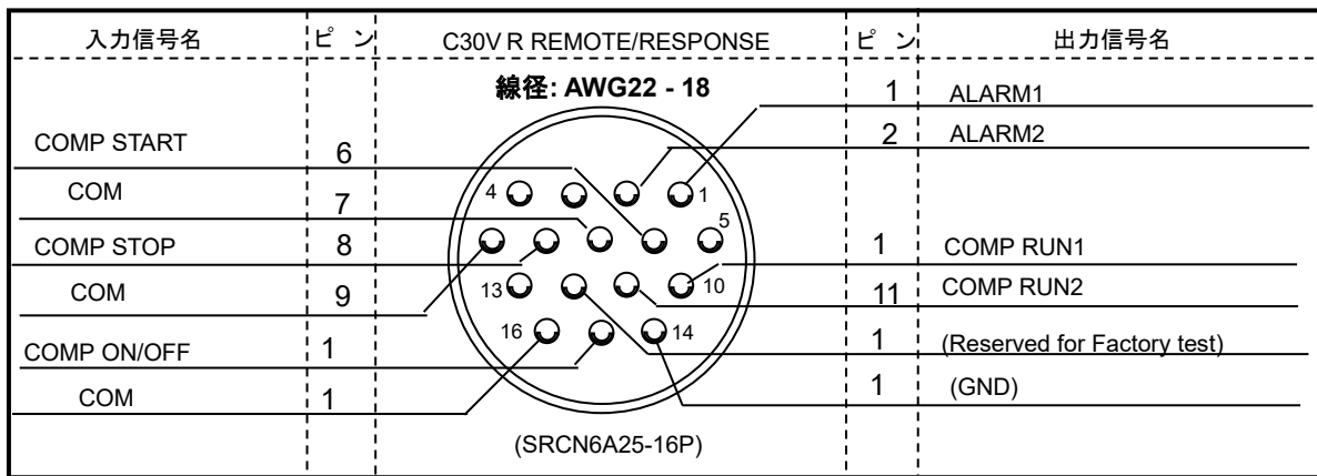
図 4-8 C30VR 用リモートコネクタピン定義(プラグ半田付け側から見て)
