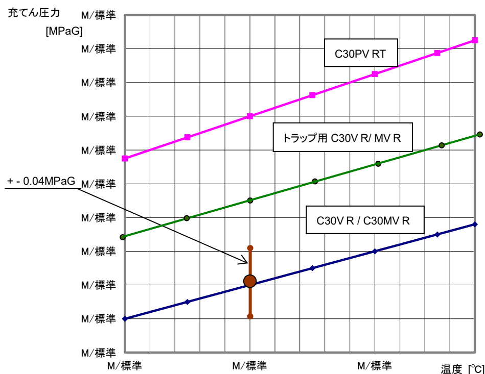
図 5-1 停止時ヘリウム充てん圧力と周囲温度
