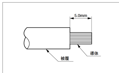
図 4-13 電線被覆剥き寸法
