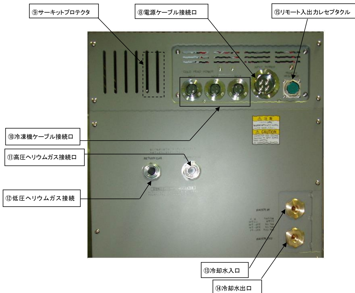
図 1-7 コンプレッサ背面
