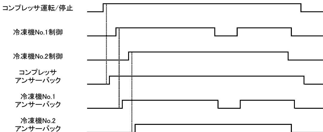
図 2-7 2台の冷凍機を「オールタネート操作モード」で運転する場合のタイムチャート
