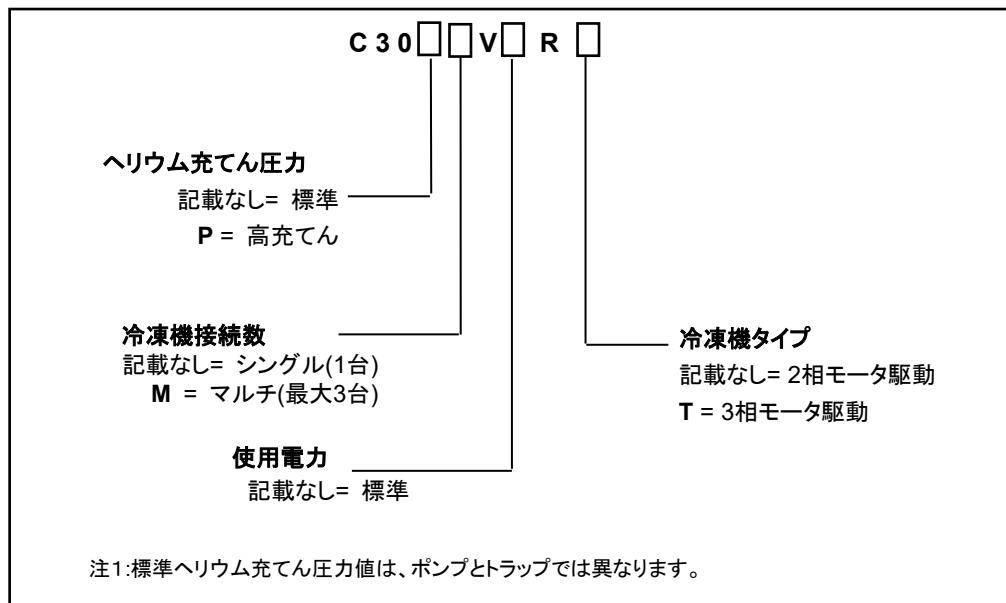
図 1-1 C30VR コンプレッサ型式
